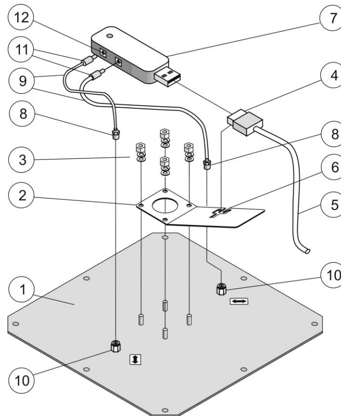
Рисунок 2. Сборка антенны
