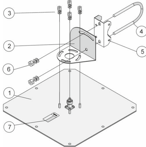
Рисунок 1 - Сборка антенны
