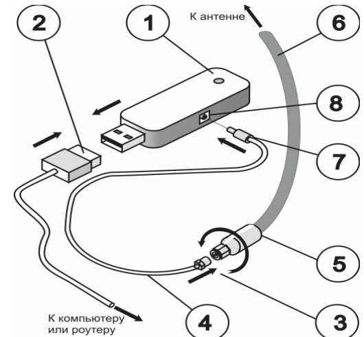
Рисунок 2 - Подключение модема
