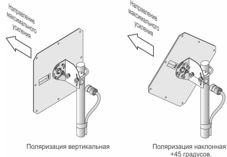
Рисунок 4 - Установка антенну на мачту. Изменение поляризации
