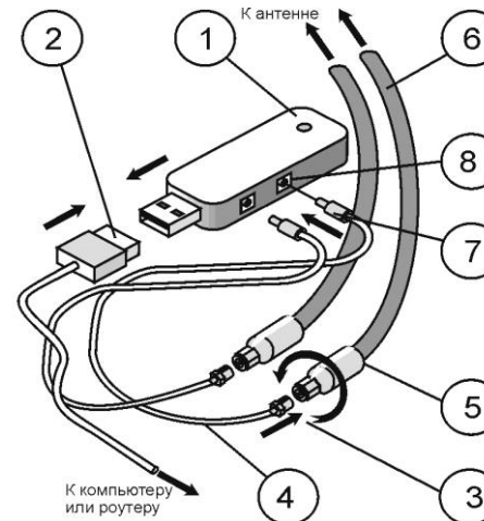
Рисунок 2 - Подключение к модему
