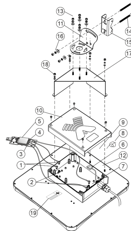
Рисунок 2. Сборка антенны
