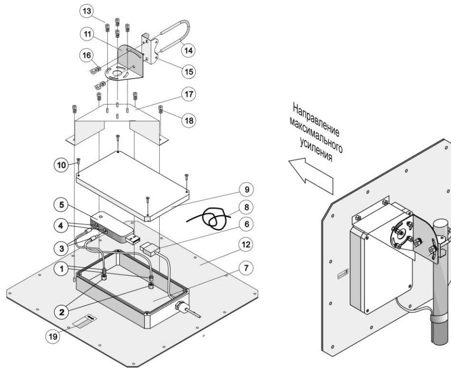
Рисунок 2. Установка антенны на мачту
