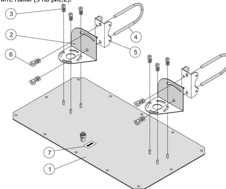
Рисунок 2. Сборка антенны на примере антенны CIFRA-12
