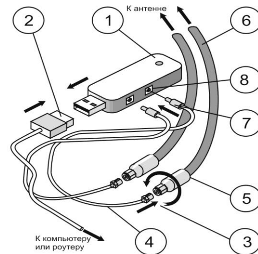
Рисунок 3 - Подключение модема
