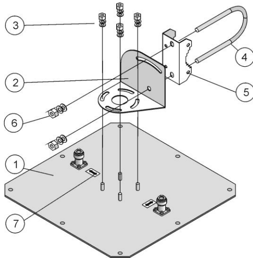
Рисунок 2 - Сборка антенны
