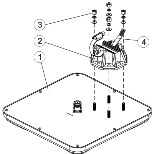
Рисунок 2 - Сборка антенны
