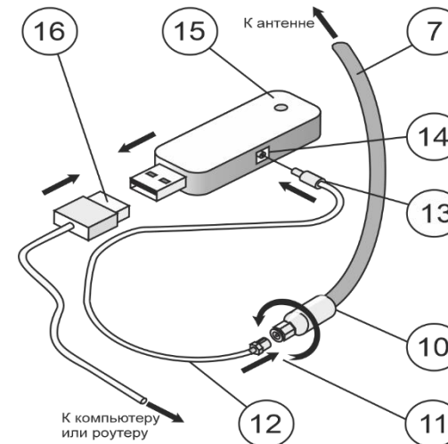
Рисунок 4 - Подключение модема
