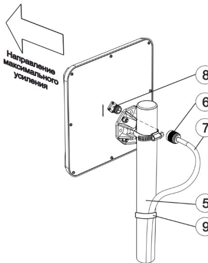
Поляризация: вертикальная
