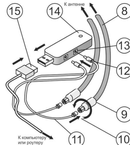
Рисунок 3 - Подключение модема
