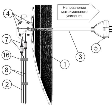
Рисунок 2 - Установка антенны на мачту
