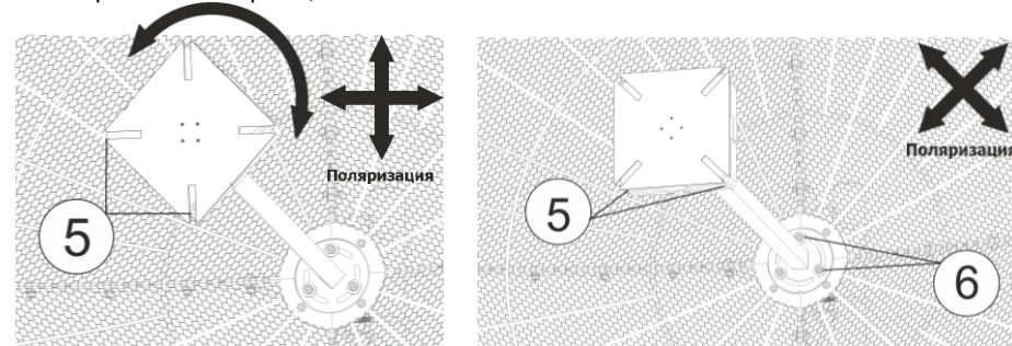
Рисунок 4 – Начальное положение облучателя с поляризацией V+H (слева, при этом более короткий кабель облучателя соответствует вертикальной поляризации, а более длинный - горизонтальной) и X-pol (справа)
