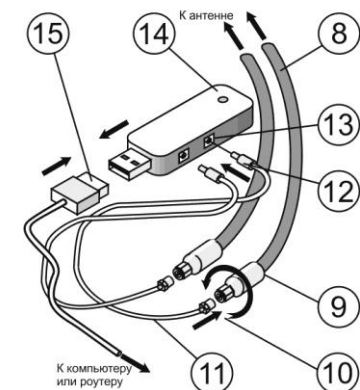
Рисунок 3 - Подключение модема
