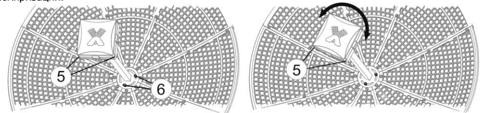
Рисунок 4 – Начальное положение облучателя с поляризацией X-pol (слева) и V+N (справа, при этом более короткий кабель облучателя соответствует вертикальной поляризации, а более длинный - горизонтальной)
