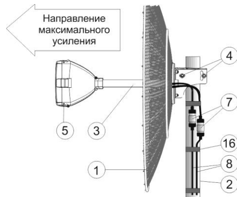
Рисунок 2 - Установка антенны на мачту
