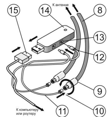
Рисунок 3 - Подключение модема
