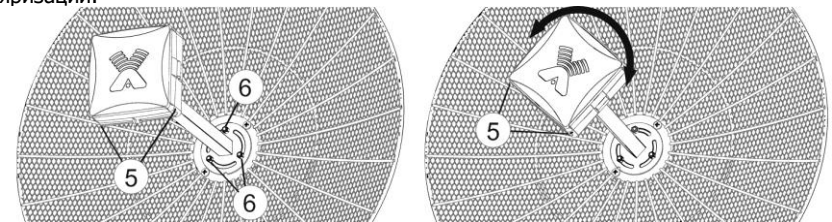
Рисунок 4 – Начальное положение облучателя с поляризацией V+H (слева, при этом более короткий кабель облучателя соответствует вертикальной поляризации, а более длинный - горизонтальной) и X-pol (справа)
