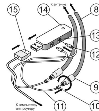
Рисунок 3 - Подключение модема
